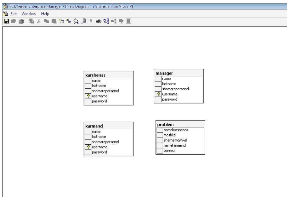
شکل ۴-۵- دیاگرام جداول
